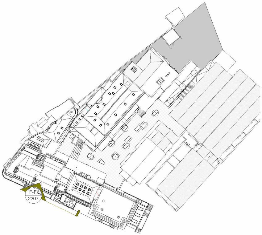
Key plan - Section F-F 1 : 1000
