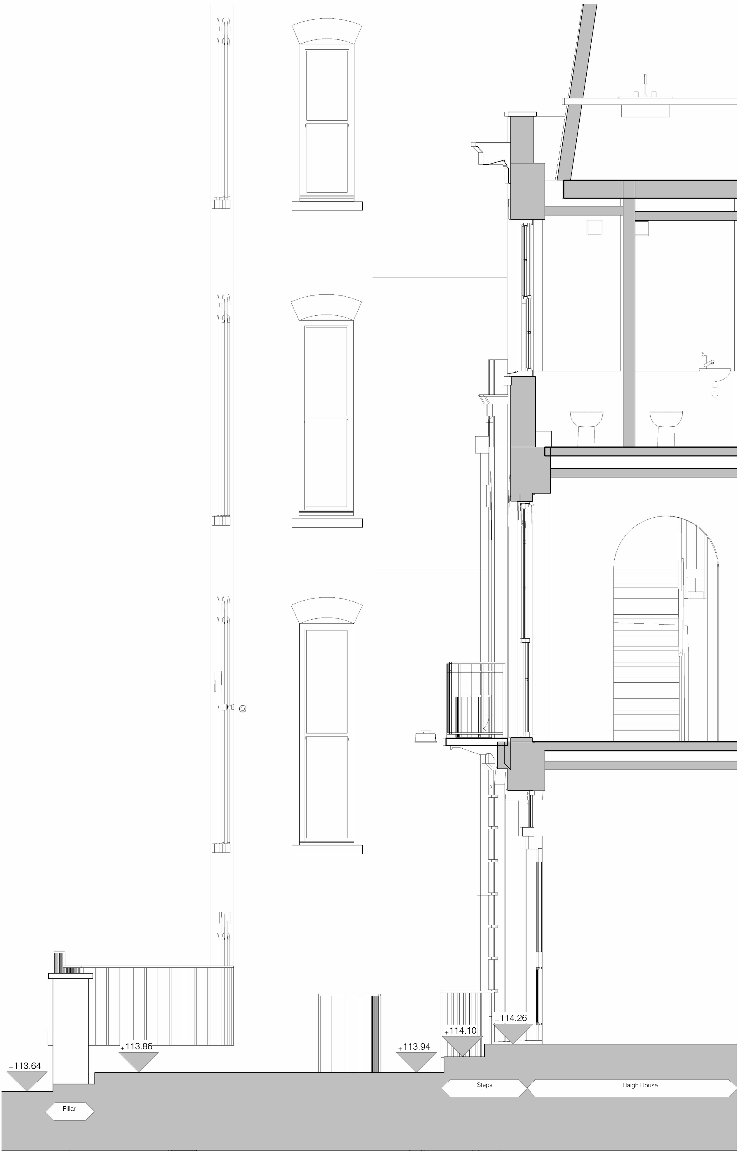
Existing Site Section E-E 1 : 25
