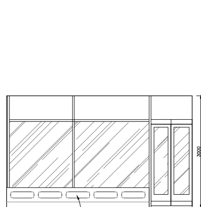
Elevation I
