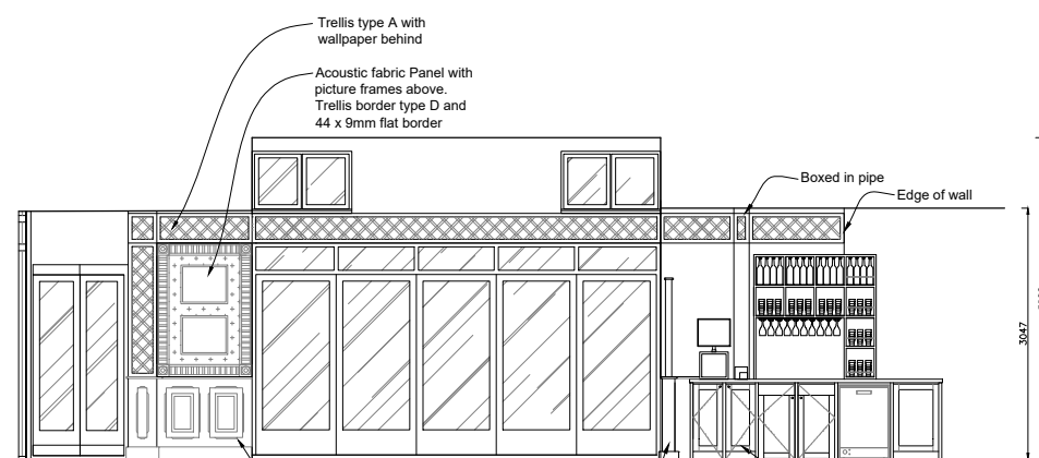
Elevation J
