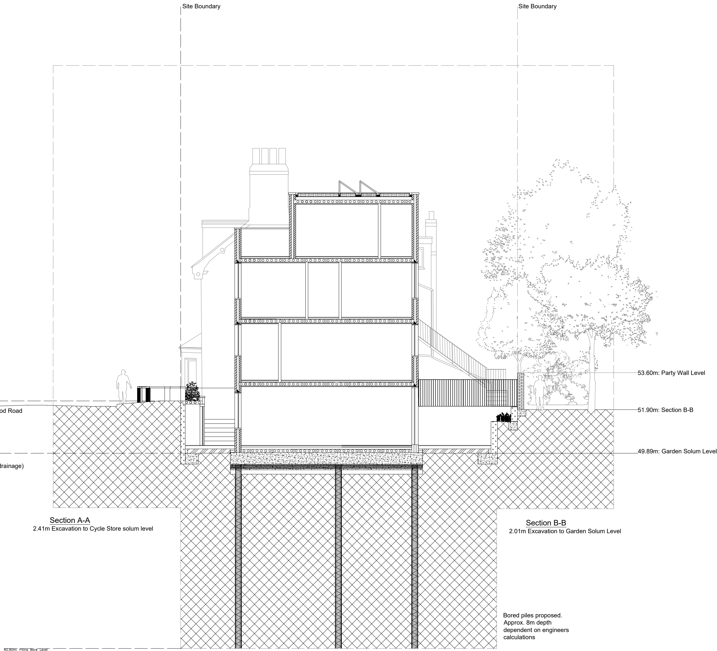
Longitudinal Section
