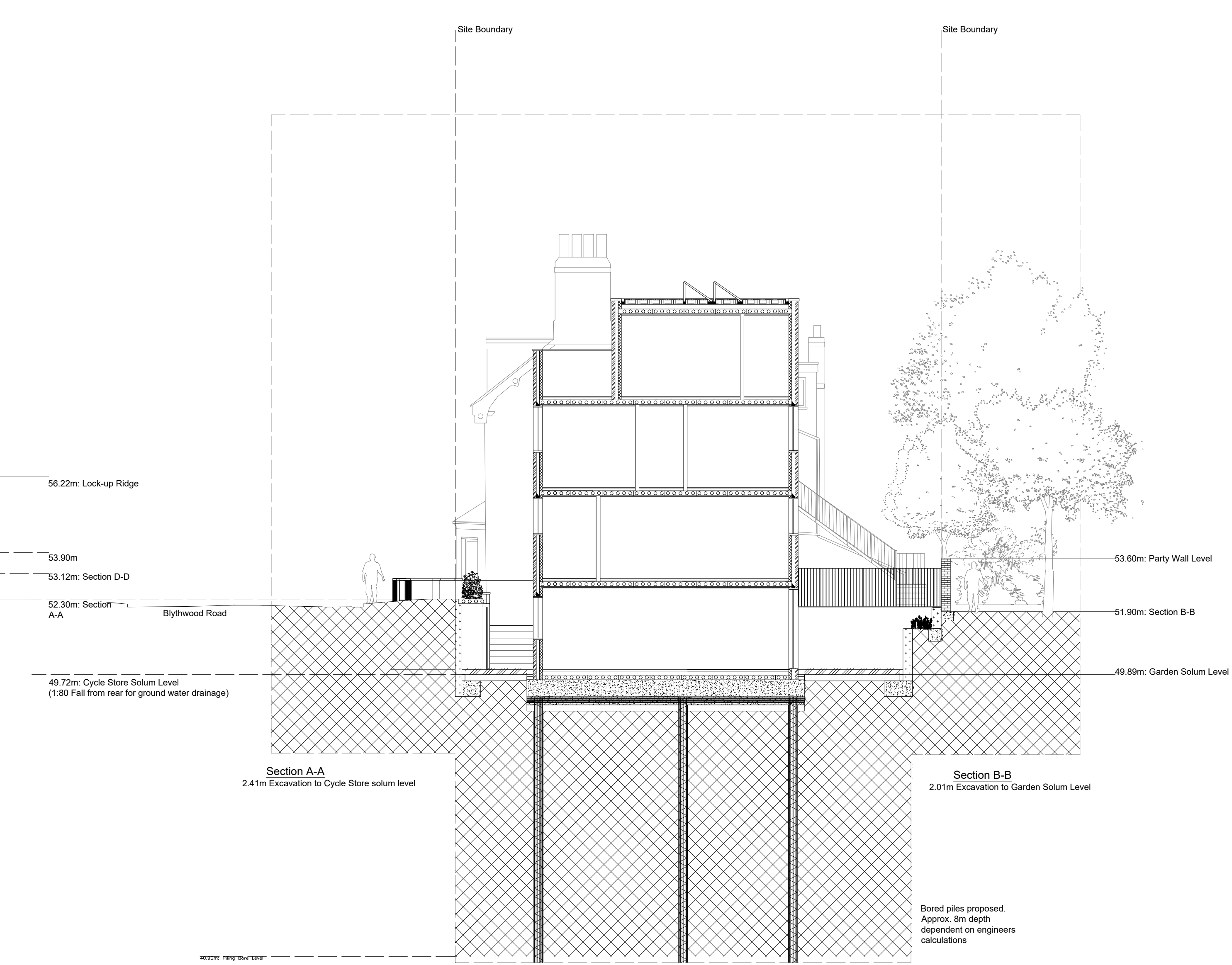
Longitudinal Section
