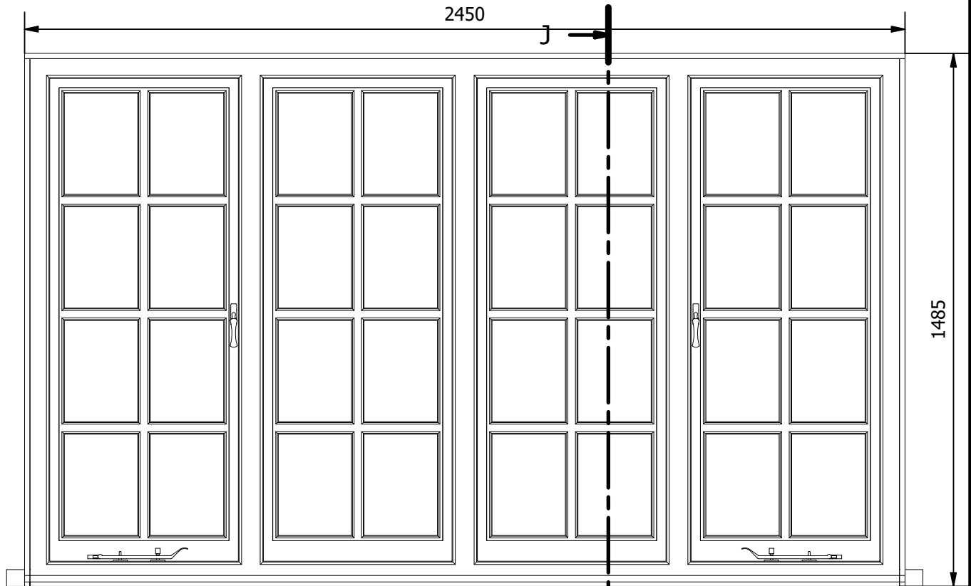
elevation section J-J ( 1 : 15 )
