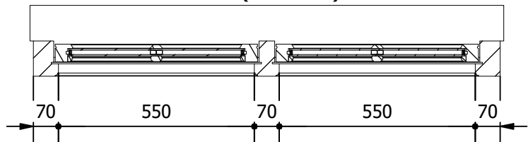
plan section B-B ( 1 : 15 )
