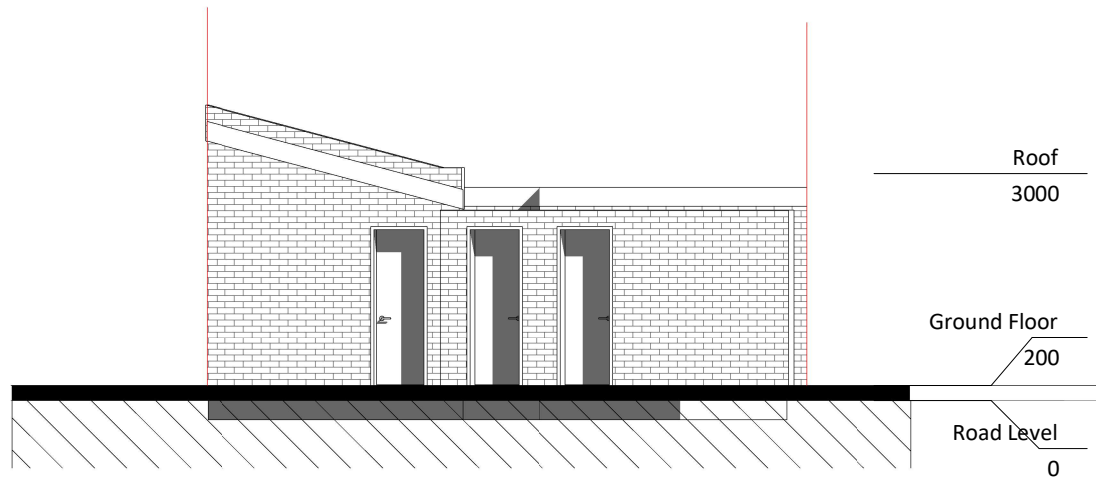
① Front 1 : 100
