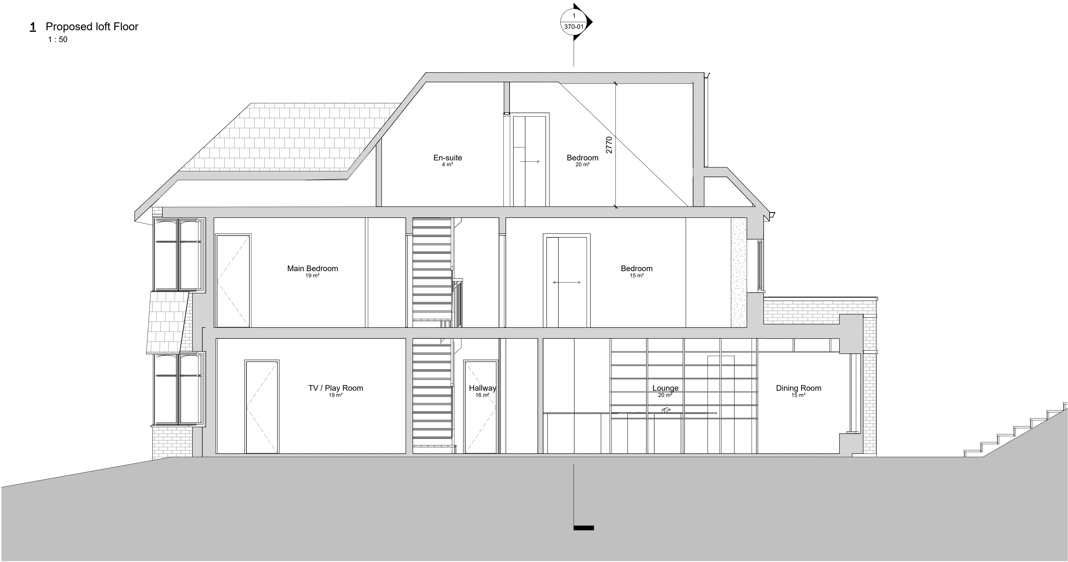
3 Loft section 1 : 50
