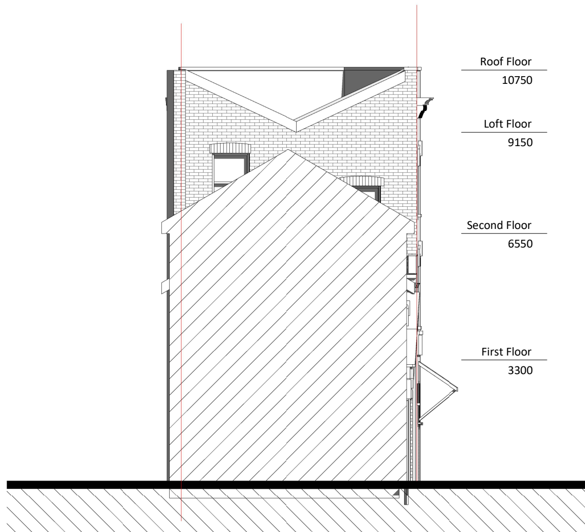
2 Rear 1 : 100
