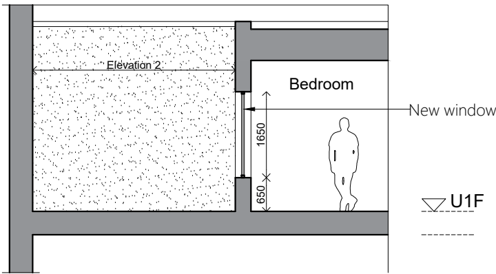
Elevation 2
