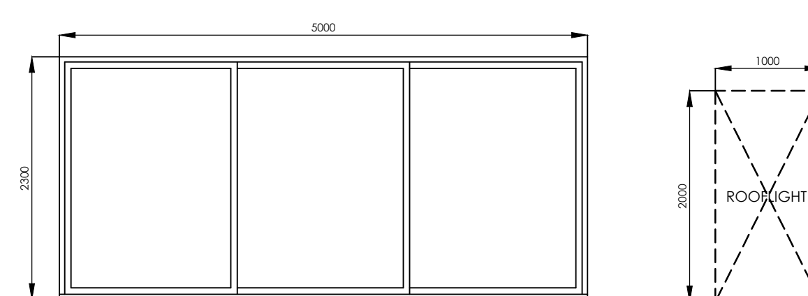
DOOR DETAILS
