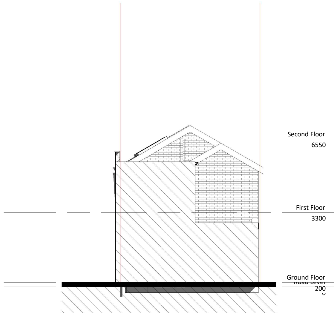
1 Front 1 : 100
