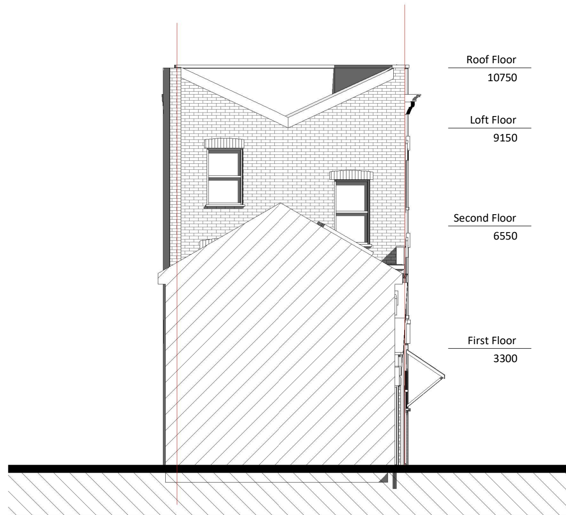
2 Rear 1 : 100
