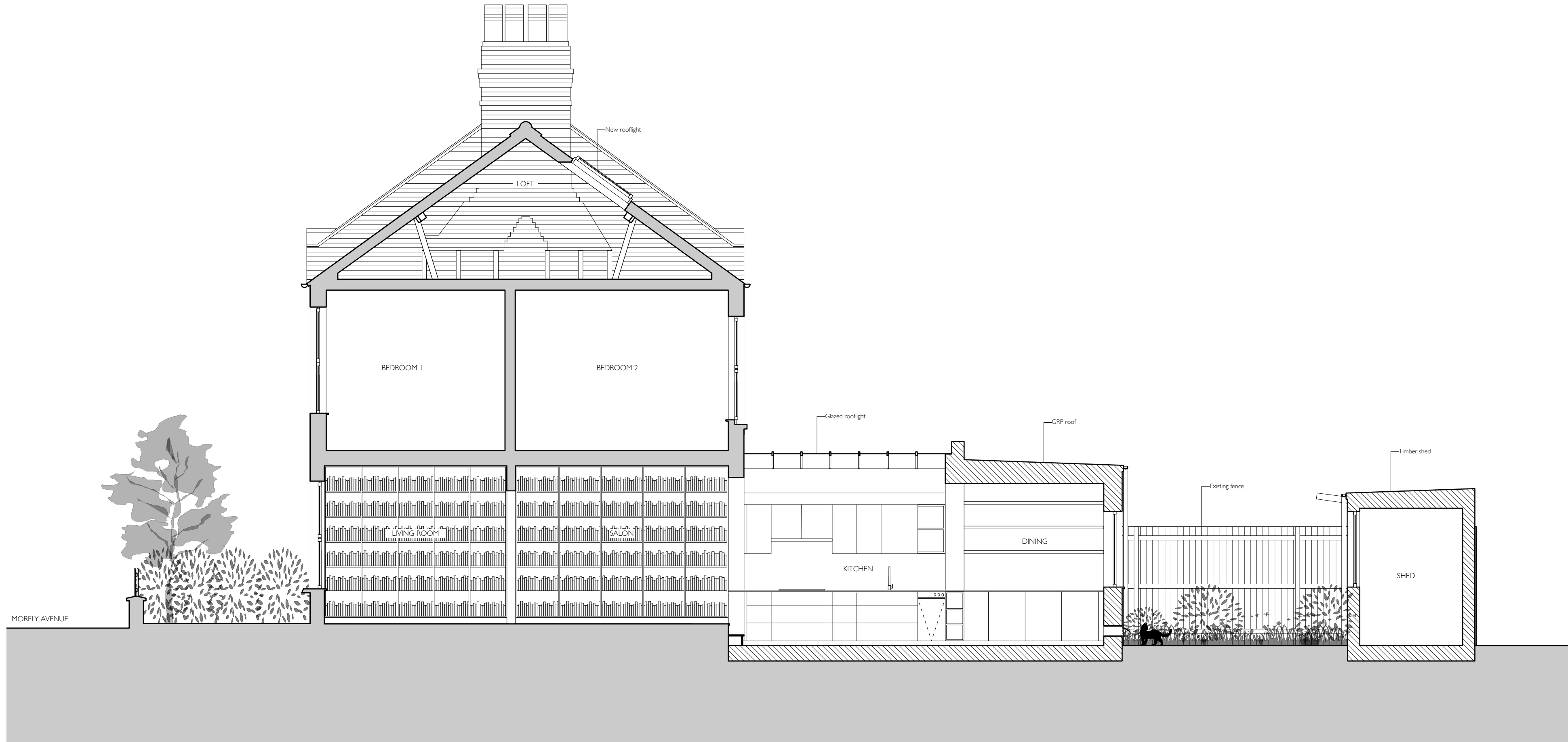
1 SECTION A 1:50 @ A1
