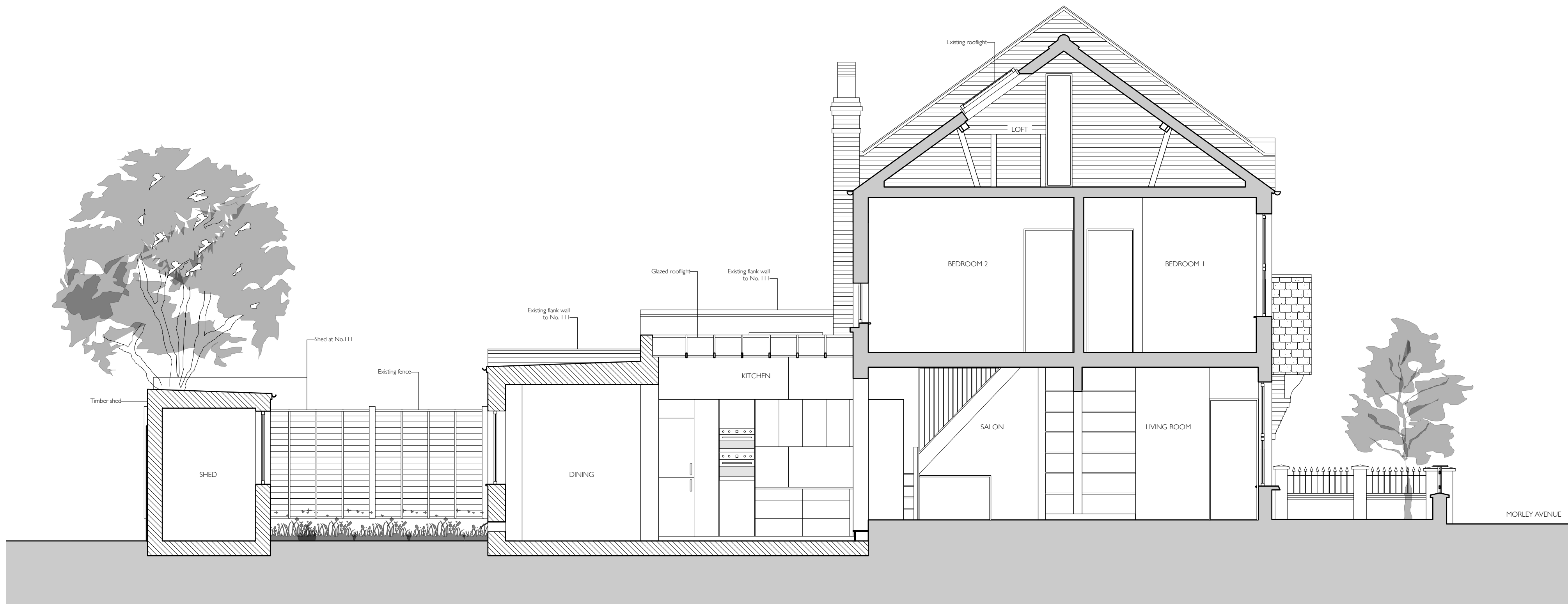
2 SECTION B 1:50 @ A1
