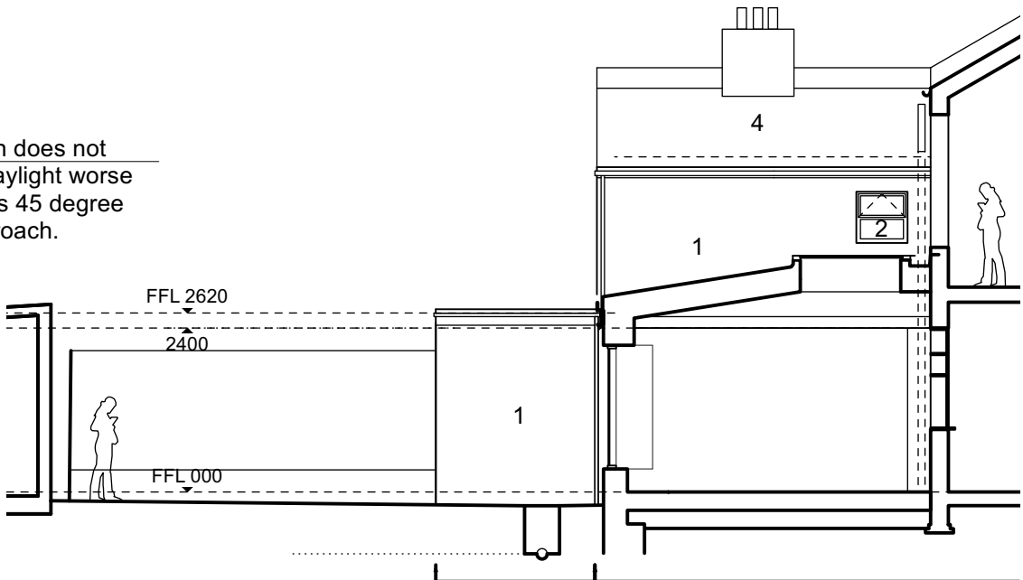
02 054 SECTION D-D
