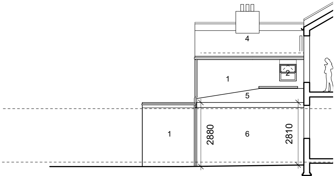
03 054 ELEVATION SIDE
