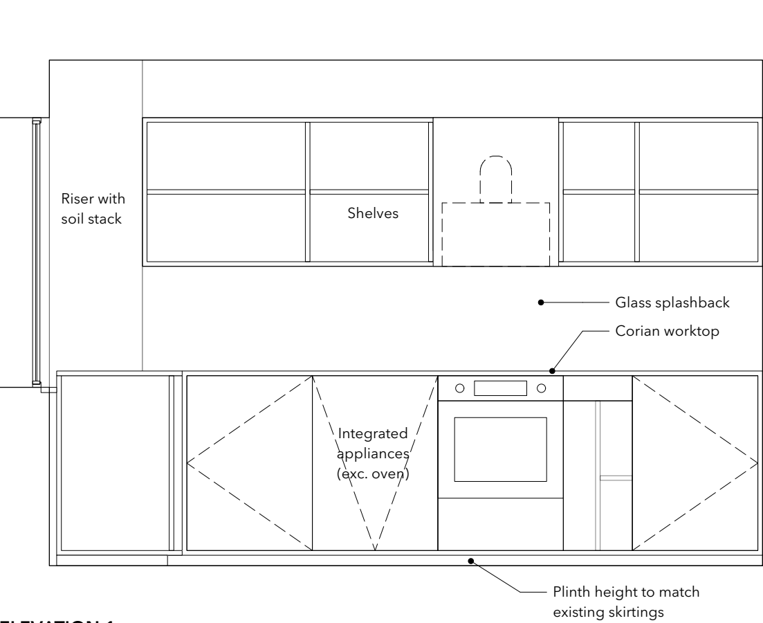
ELEVATION 1
