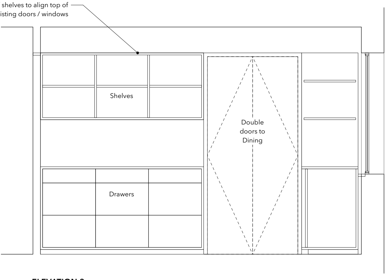
ELEVATION 2
