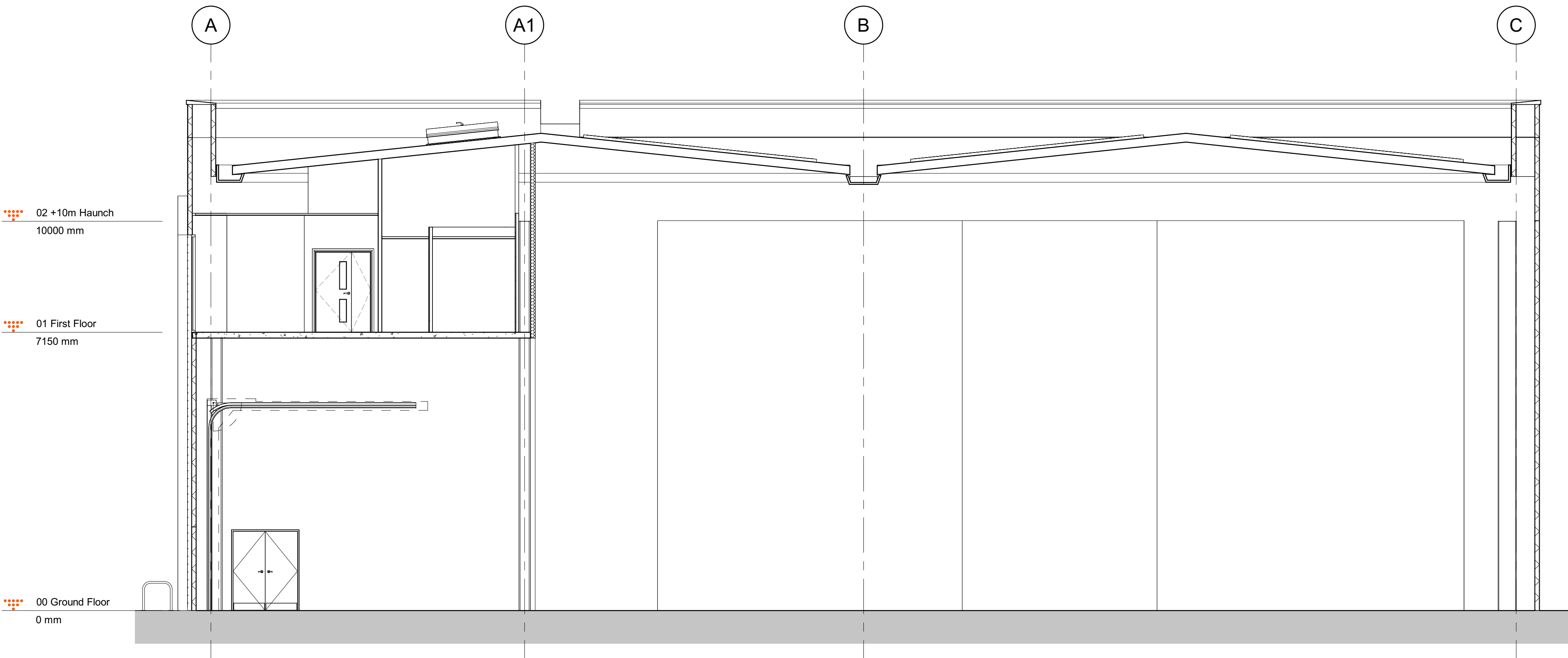
1 Warehouse Section 1 1 : 75
