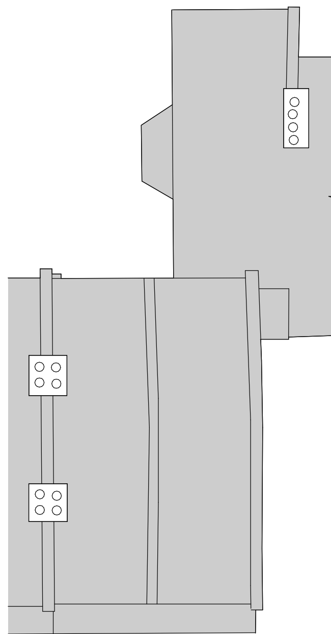
3 PL000 - Existing Roof Plan 1 : 100
