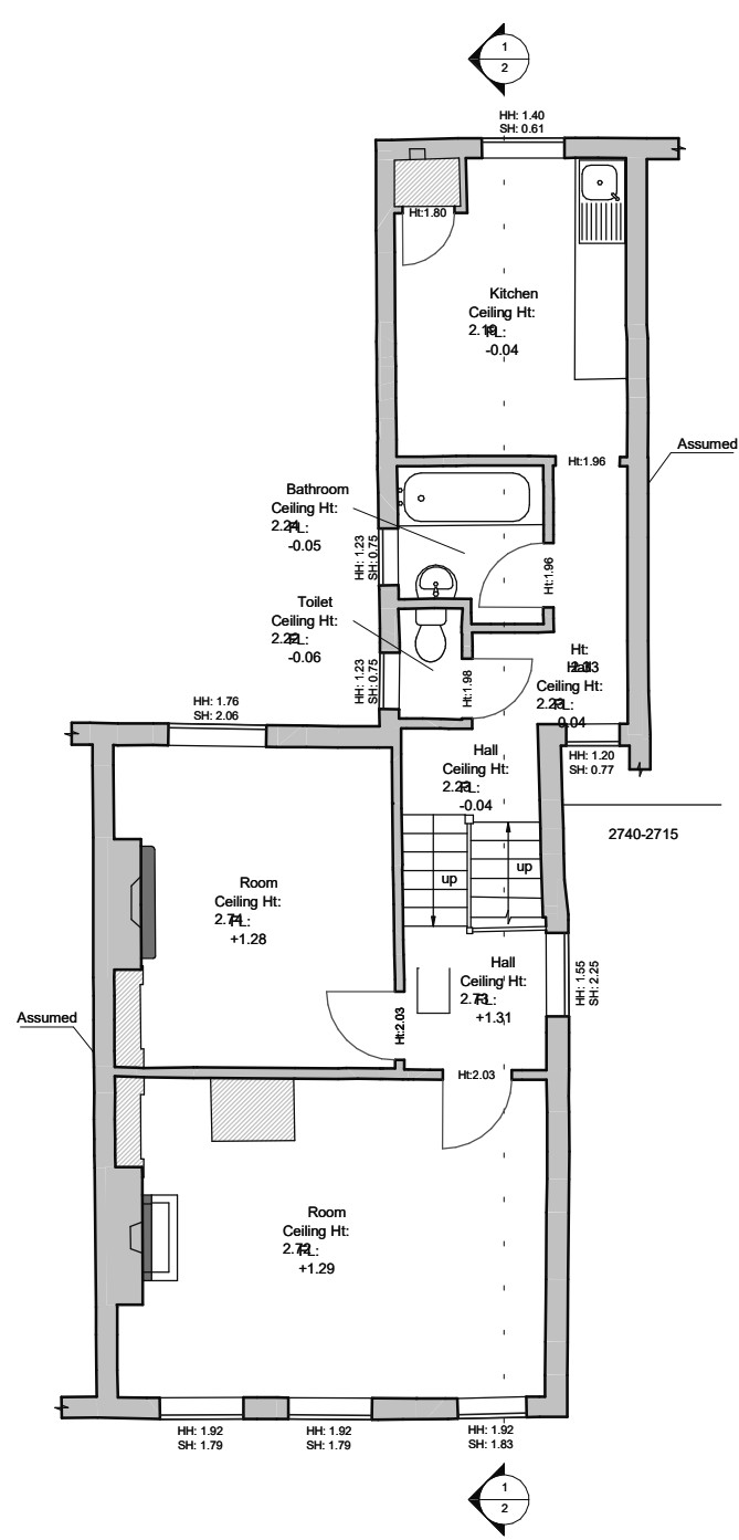
2 PL000 - Existing 1F Plan 1 : 100
