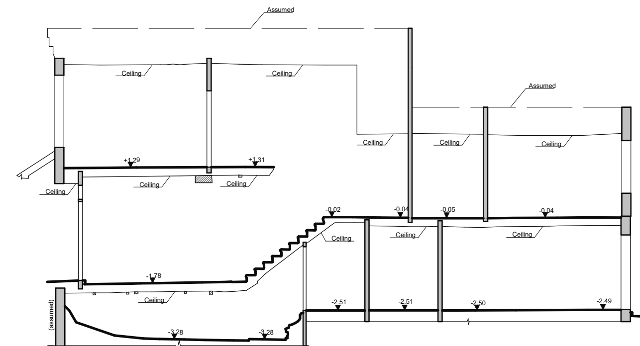
8 PL000 - Existing Section 1 1 : 100
