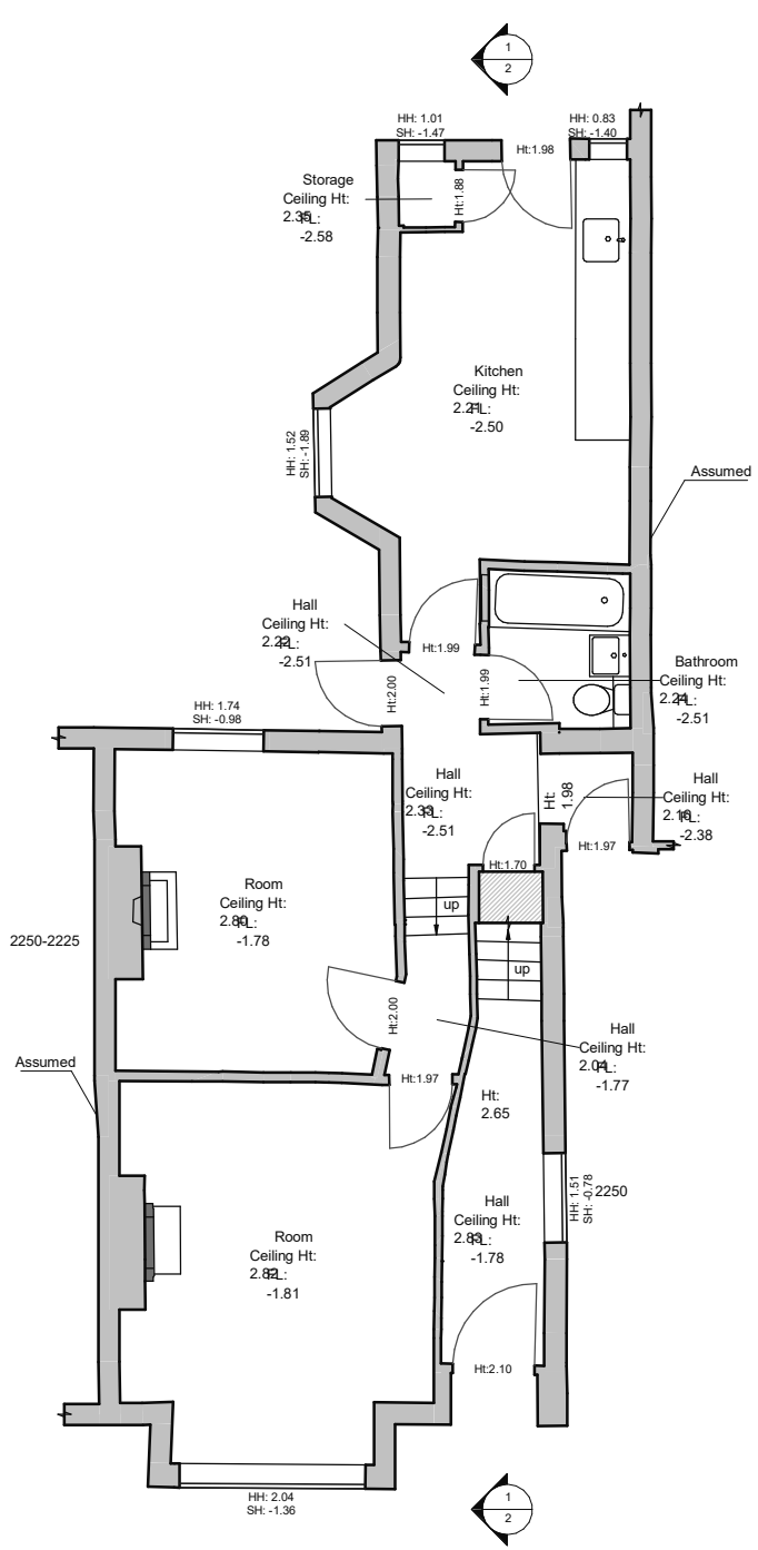
1 PL000 - Existing GF Plan 1 : 100
