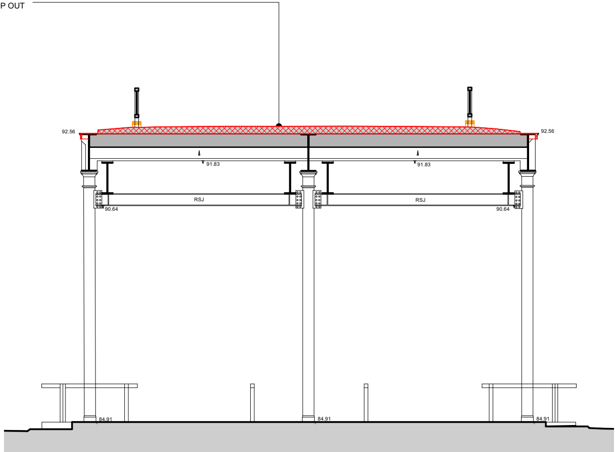
2 STRIP OUT SECTION D Scale: 1:100
