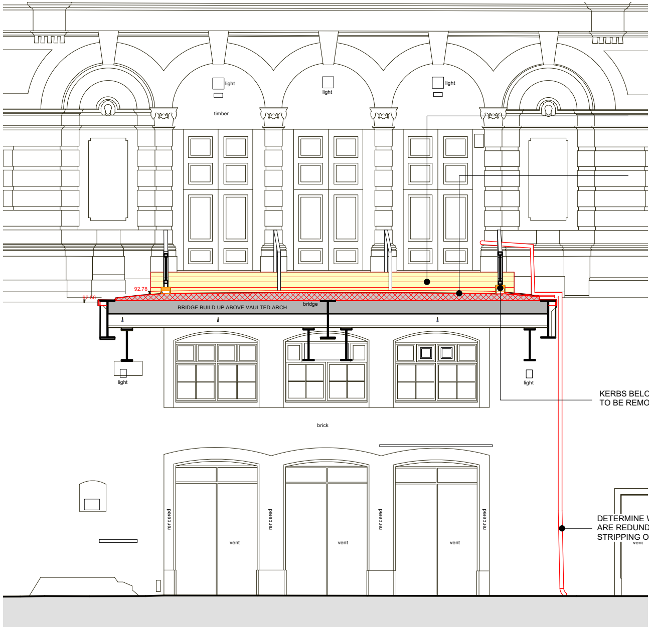
1 STRIP OUT SECTION A Scale: 1:100
